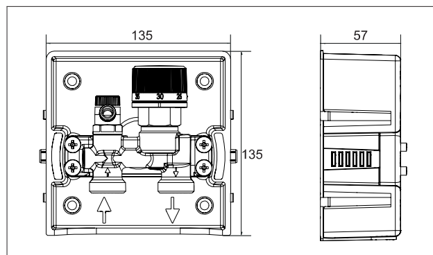
Рис. 3: Габаритные размеры в мм
